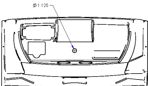
VIEW A-A
